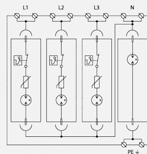
Schéma zapojení
