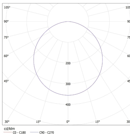
MILED0 (kat 31075) SP LED N 6W NW-S / LDC (Polar)
